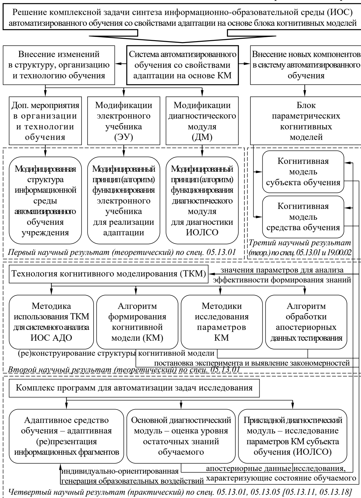
Рисунок 3.2. Комплексный подход к синтезу и системному анализу информационно-образовательной среды системы автоматизированного (дистанционного) обучения с элементами адаптации на основе блока параметрических когнитивных моделей
