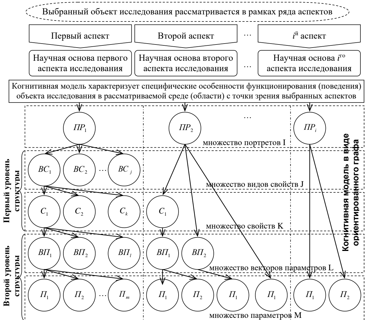
Рисунок 3.4. Рекомендуемая основа для построения структуры когнитивной модели (формальное представление)
