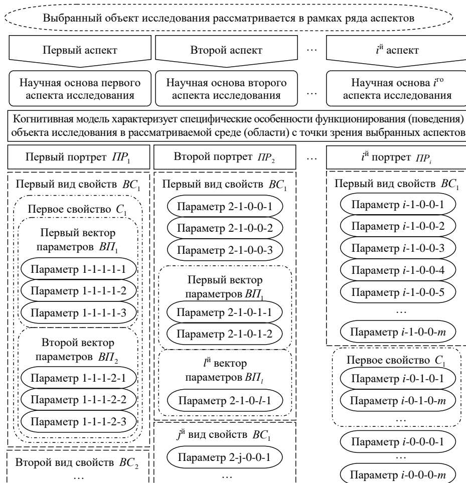
Рисунок 3.5. Рекомендуемая основа для построения структуры когнитивной модели (неформальное представление)
