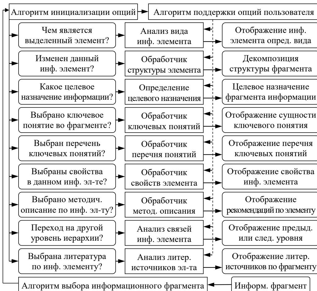
Рисунок 2.11. Алгоритм обработки событий, инициируемых пользователем в адаптивном средстве обучения
