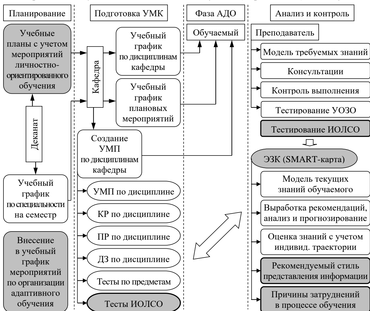
Рисунок 2.3. Модификации в технологическом процессе формирования знаний при реализации лично-ориентированного (адаптивного) автоматизированного (дистанционного) обучения
