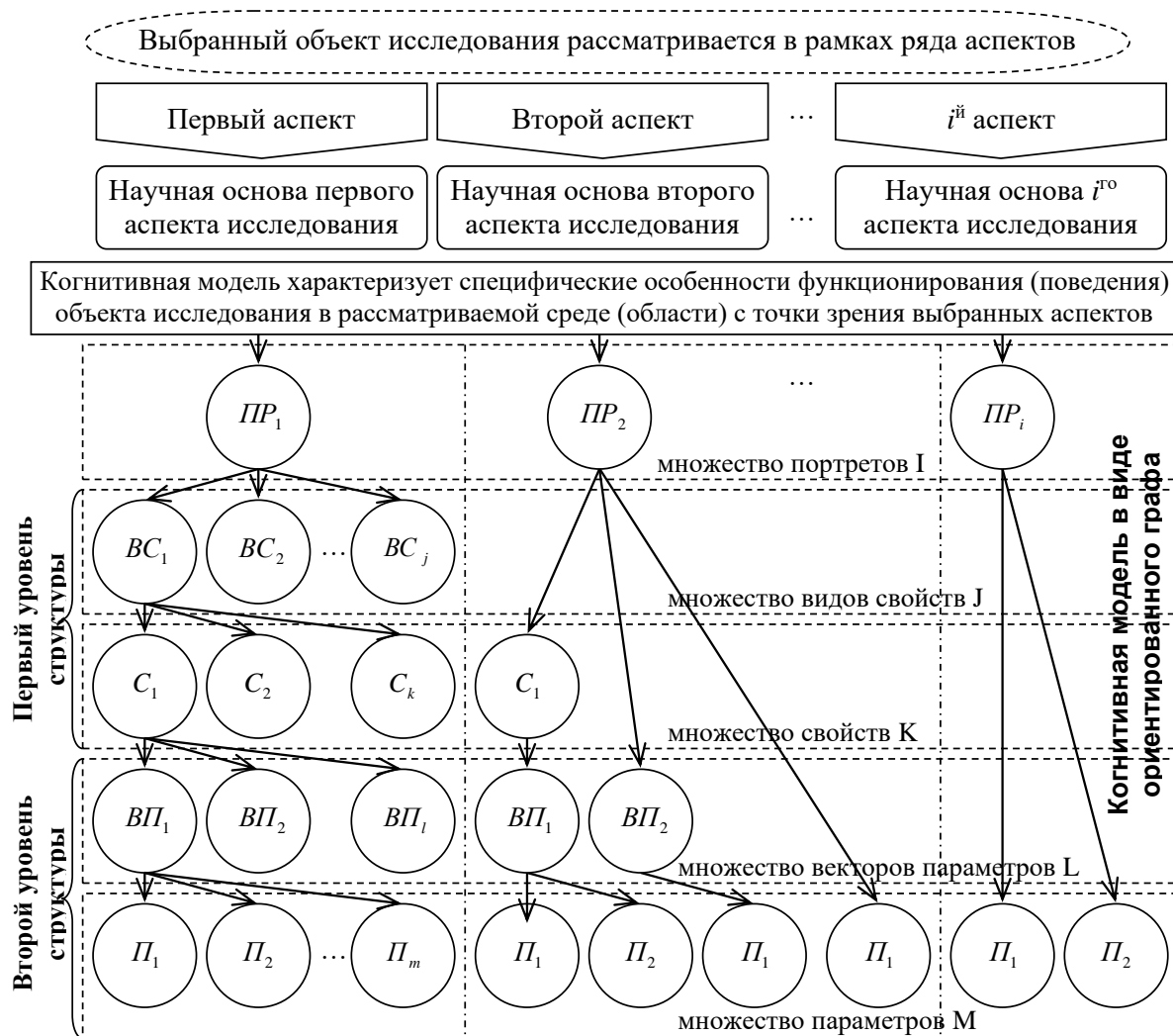
Рисунок 3.4. Рекомендуемая основа для формирования структуры когнитивной модели (формальное представление)
