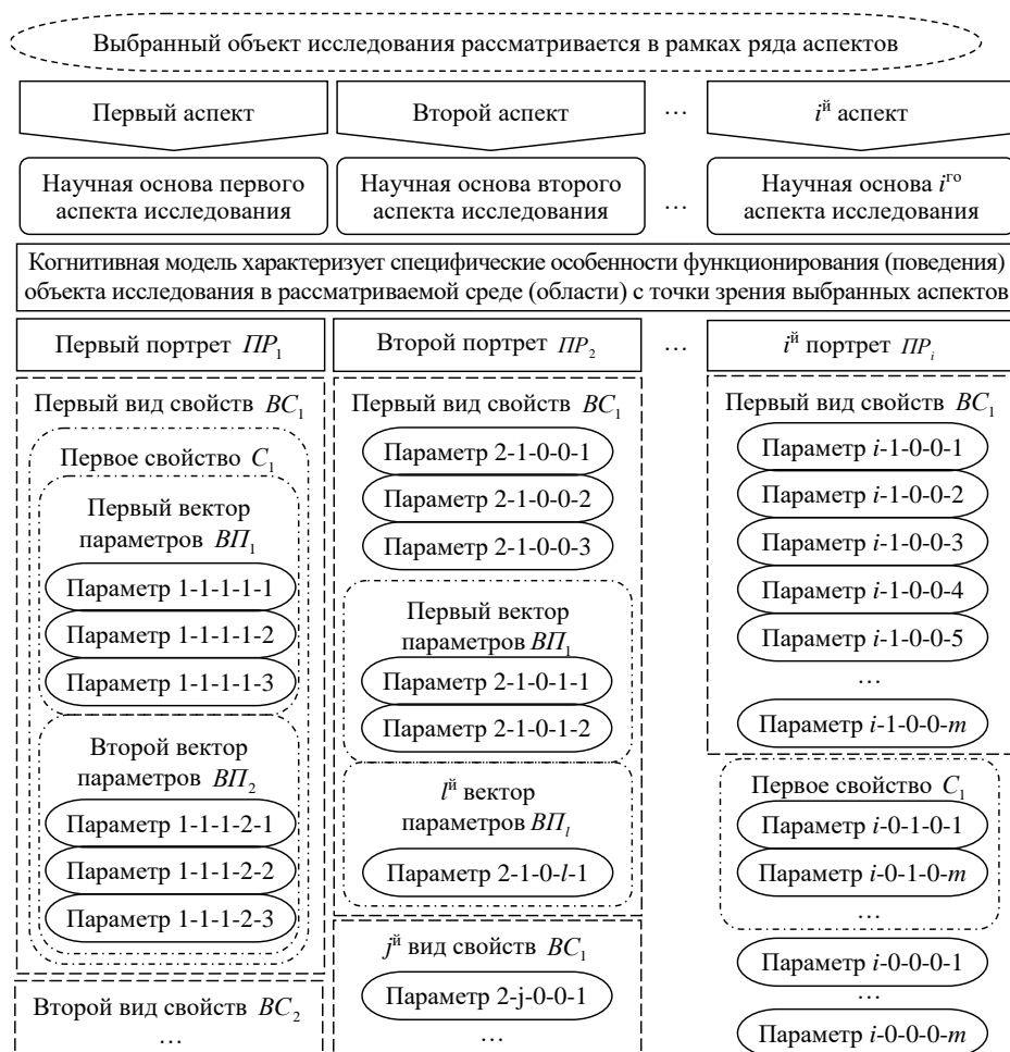
Рисунок 3.5. Рекомендуемая основа для формирования структуры когнитивной модели (неформальное представление)
